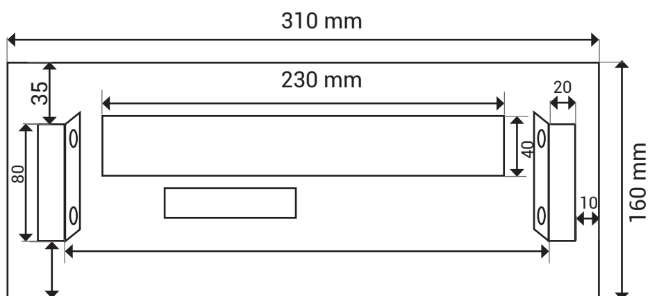
Rückansicht
